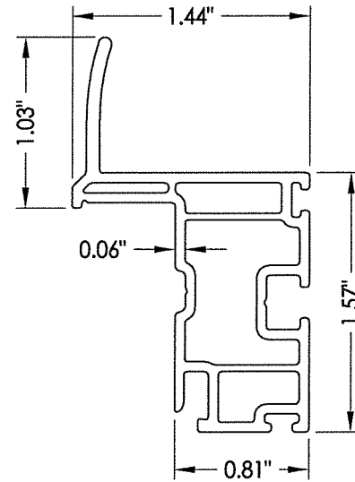
8 HANDLE STILE
